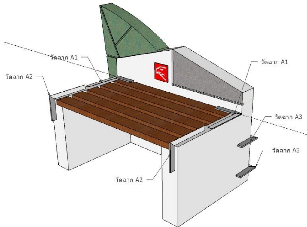
แสดงจุดวัดมิติ ด้านฉาก
