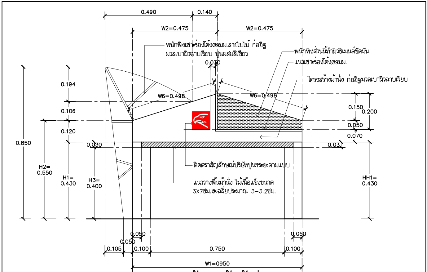
รูปด้านหน้าม้านั่ง-1 มาตราส่วน 12.5
