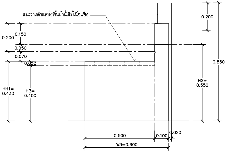
รูปด้านข้างม้านั่ง-2 มาตราส่วน 12.5
