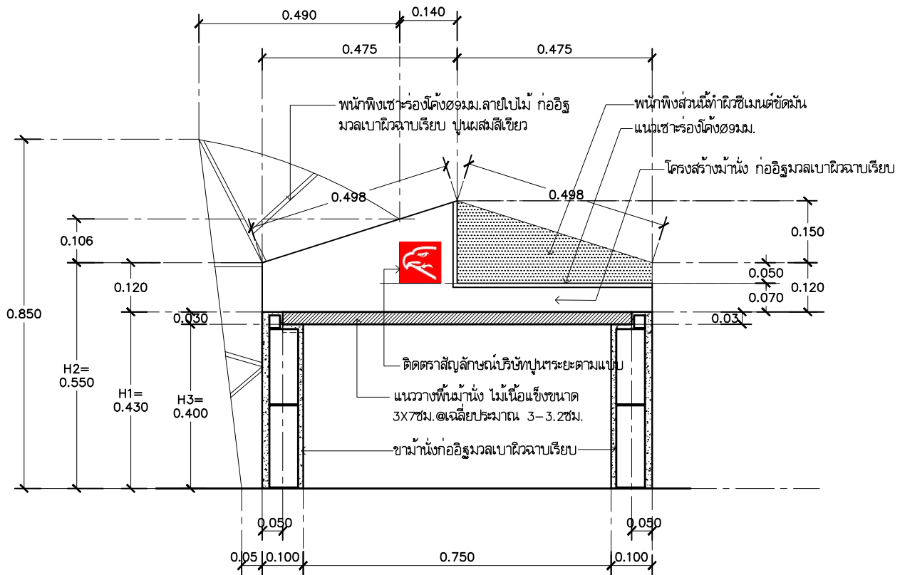
รูปตัดม้านั่ง A-A มาตราส่วน 12.5
