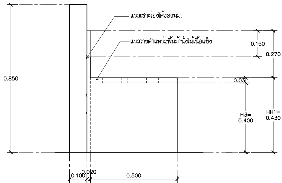
รูปด้านข้างม้านั่ง-4 มาตราส่วน 12.5
