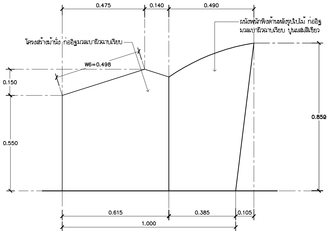
รูปด้านหลังม้านั่ง-3 มาตราส่วน 12.5
