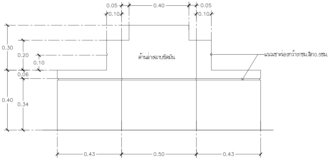
รูปด้านข้างมานั่งหินขัด-3 มาตราส่วน 12.5
