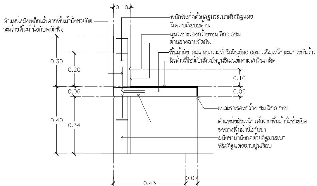
รูปตัดแนว A-A มาตราส่วน 12.5
