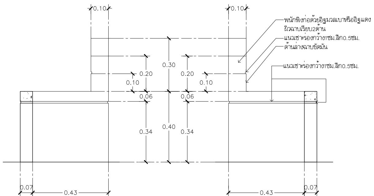
รูปด้านข้างมานั่งหินขัด-2 มาตราส่วน 12.5
