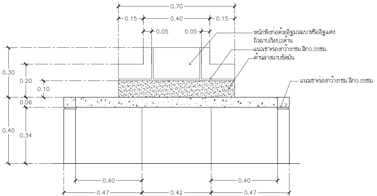
รูปด้านหน้ามานั่งหินขัด-1 มาตราส่วน 12.5
