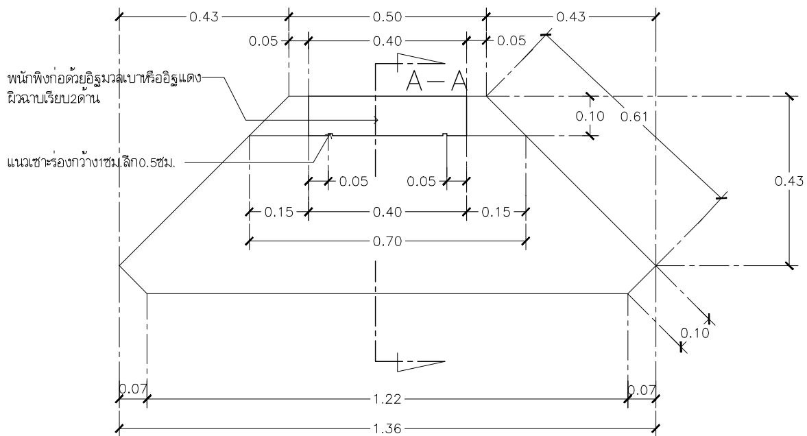
แบบผังแสดงพนักรังผึ้งม้านั่ง-2 มาตราส่วน 12.5
