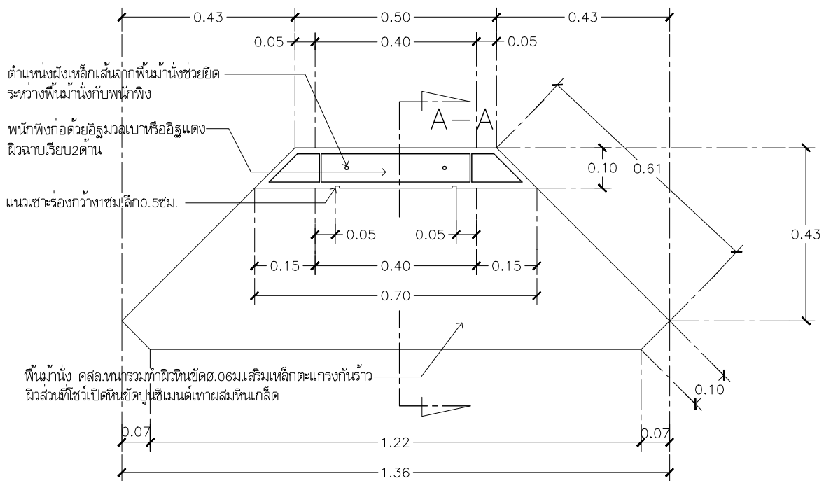
แบบผังแสดงพนักรังผึ้งม้านั่ง-1 มาตราส่วน 12.5
