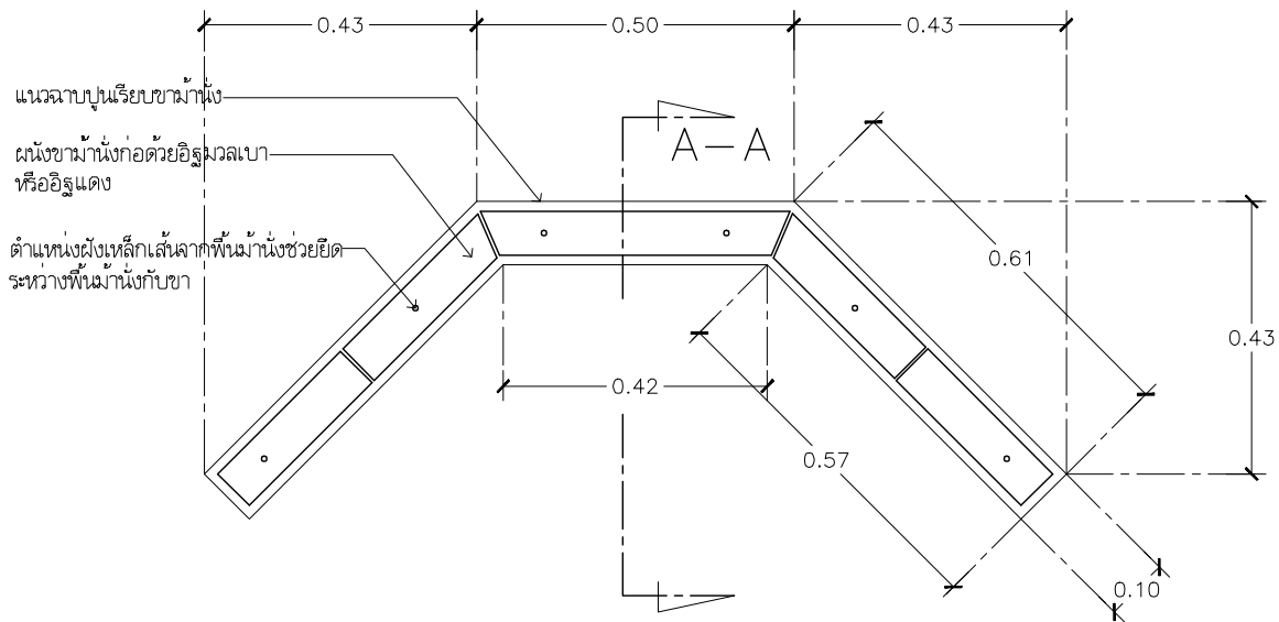
แบบผังขามานั่ง มาตราส่วน 12.5
