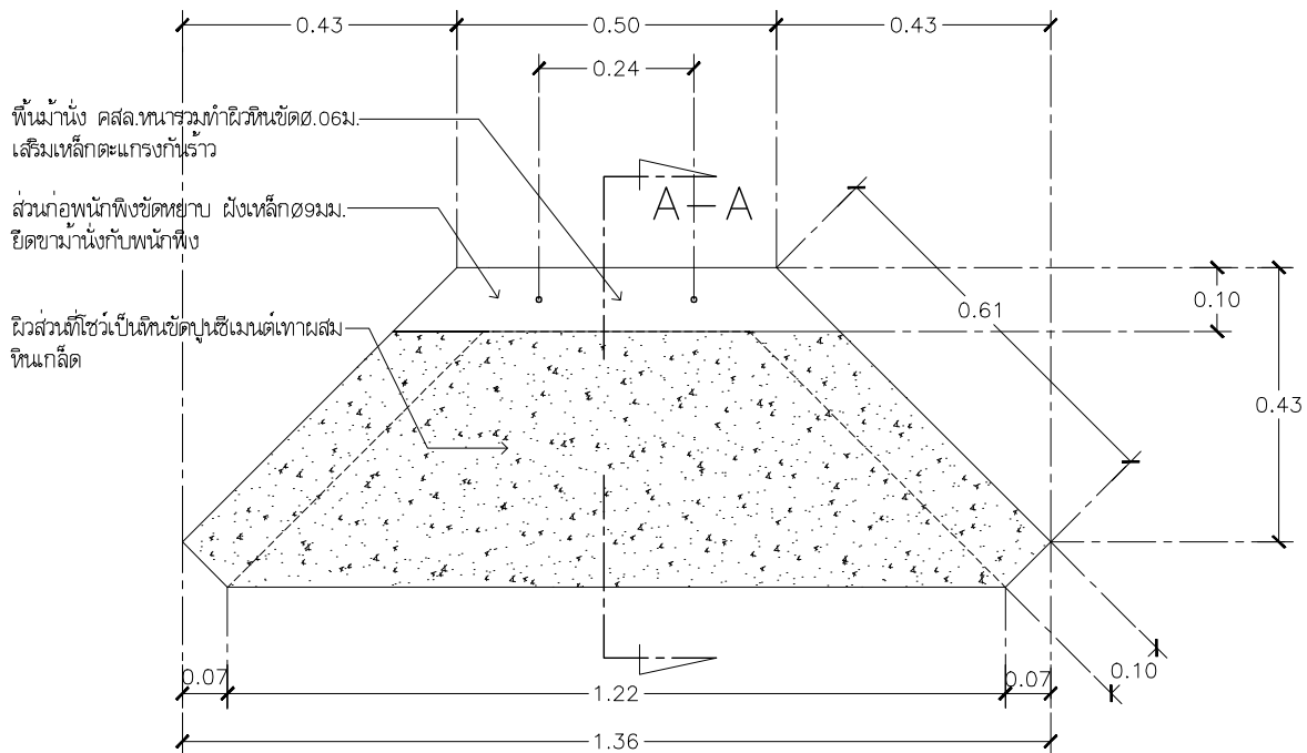
แบบแผ่นพื้นมานั่งหินขัด มาตราส่วน 12.5
